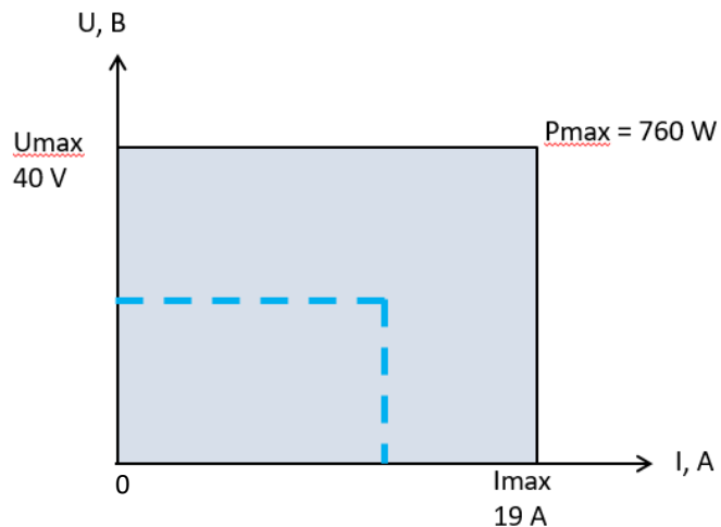
GEN40-19
